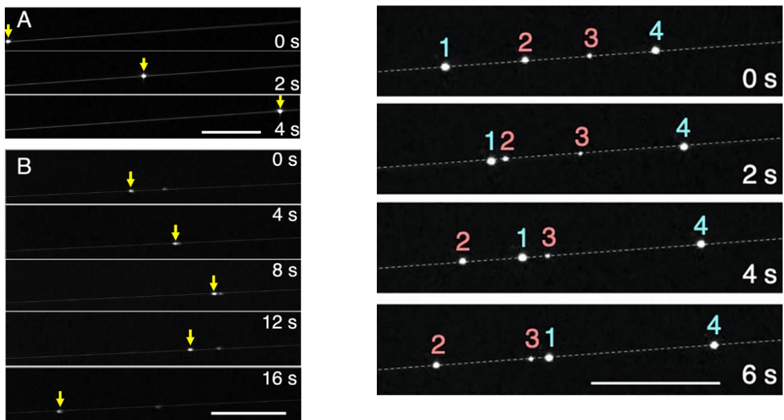
図 2. (A) 粒径 50 nm のナノダイヤモンド粒子がナノファイバーに沿って光圧輸送される様子を観測した顕微鏡画像。矢印が粒子の位置，点線がナノファイバーの位置。(B) 入射するレーザー光の強度を変化させることにより，ナノファイバー上で自在に操作する様子を観測した顕微鏡画像。 (右図) ナノダイヤモンド粒子の窒素空孔中心 (構造欠陥) の有無による光選別輸送実験 (2 秒毎の顕微鏡写真，点線がナノファイバーの位置，1 と 4 が構造欠陥含有粒子，2 と 3 は構造欠陥非含有粒子，スケールバーは 100 \mu\text{m} )。
