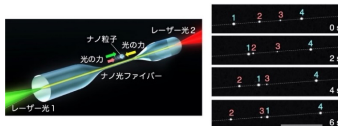
(左) ナノファイバーを用いた光の力によるナノ粒子の捕集・特性選別・分離輸送の概念図
